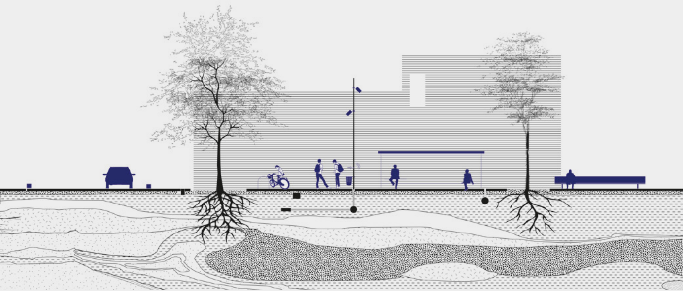
Coupe schématique dissociant les éléments de l'espace public les plus pérennes et associés au domaine du sol (en noir) et les éléments d'usage et de mobilier appelés à évoluer et être renouvelés dans un plus court terme (en bleu).
