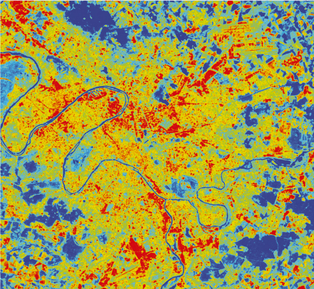
Thermographie d’été, 2019 Température au sol et sur les toits des bâtiments. Image Landsat, 20 août, 2010 38°C 25°C 15°C
